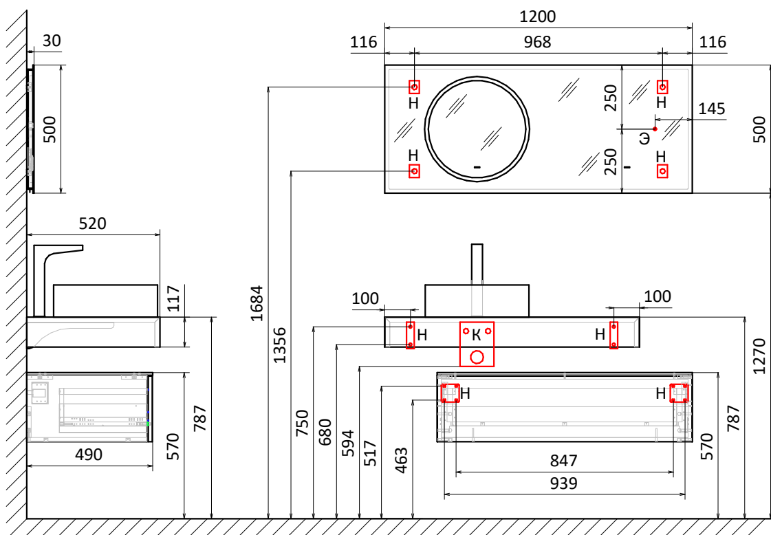
Тумба подвесная Modulare 100
