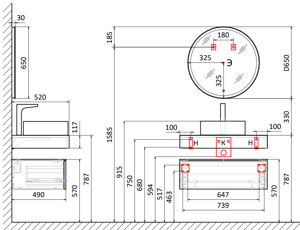
Тумба подвесная Modulare 80
